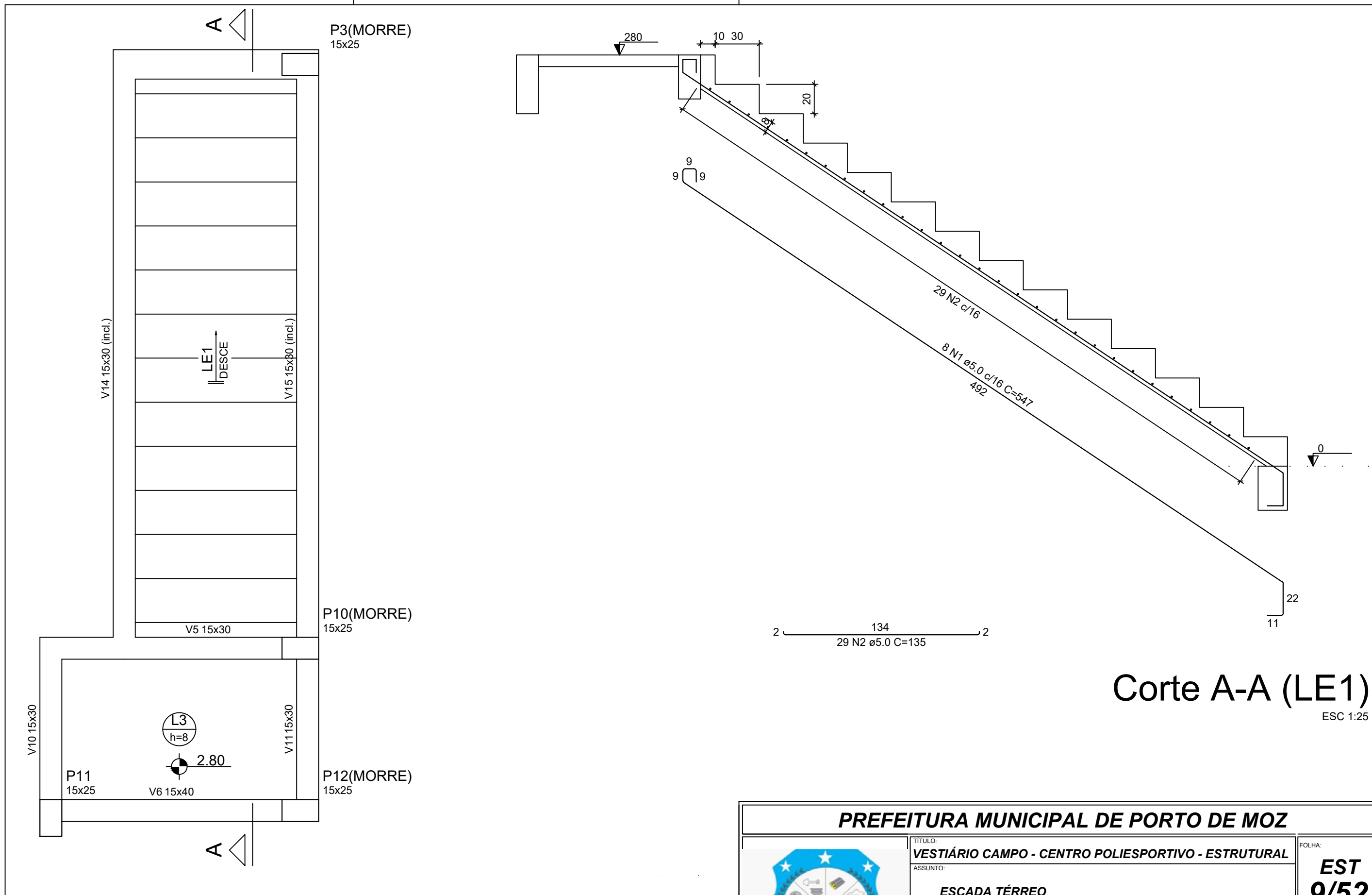
Armação positiva da escada E1 ESC 1:25
