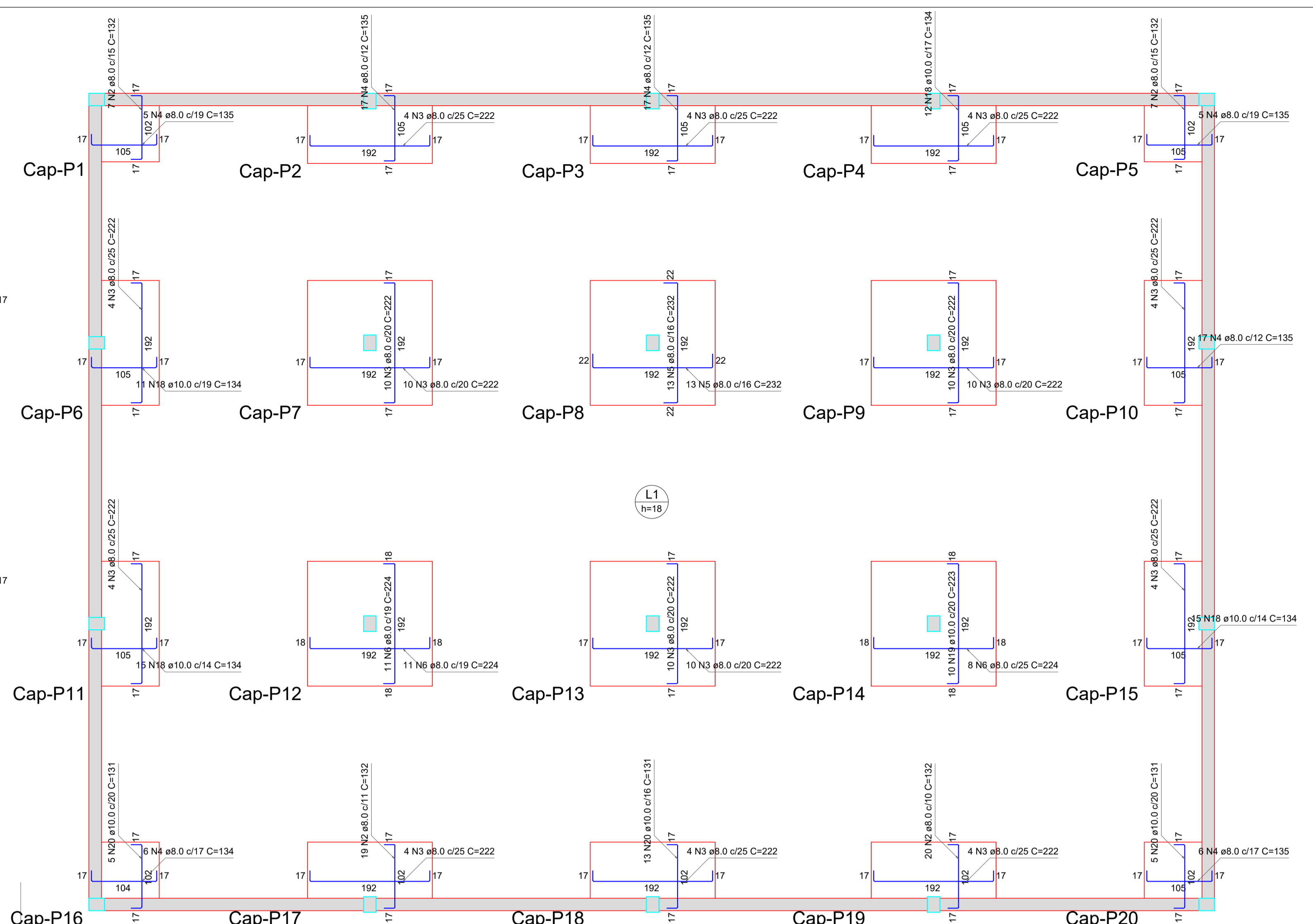
Armação positiva das regiões maciças do pavimento LAJE
