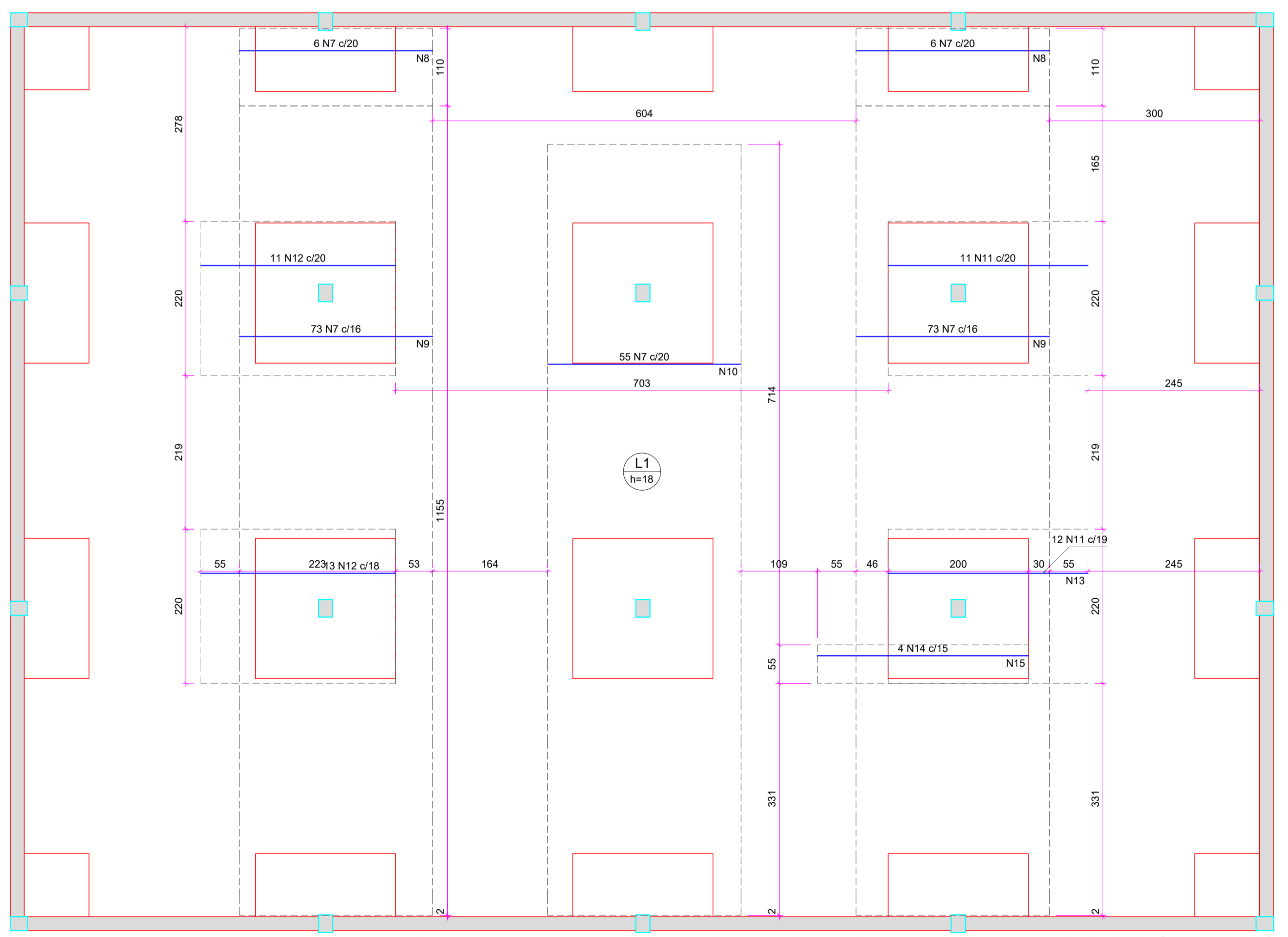
Armação negativa das lajes do pavimento LAJE (Eixo X)
