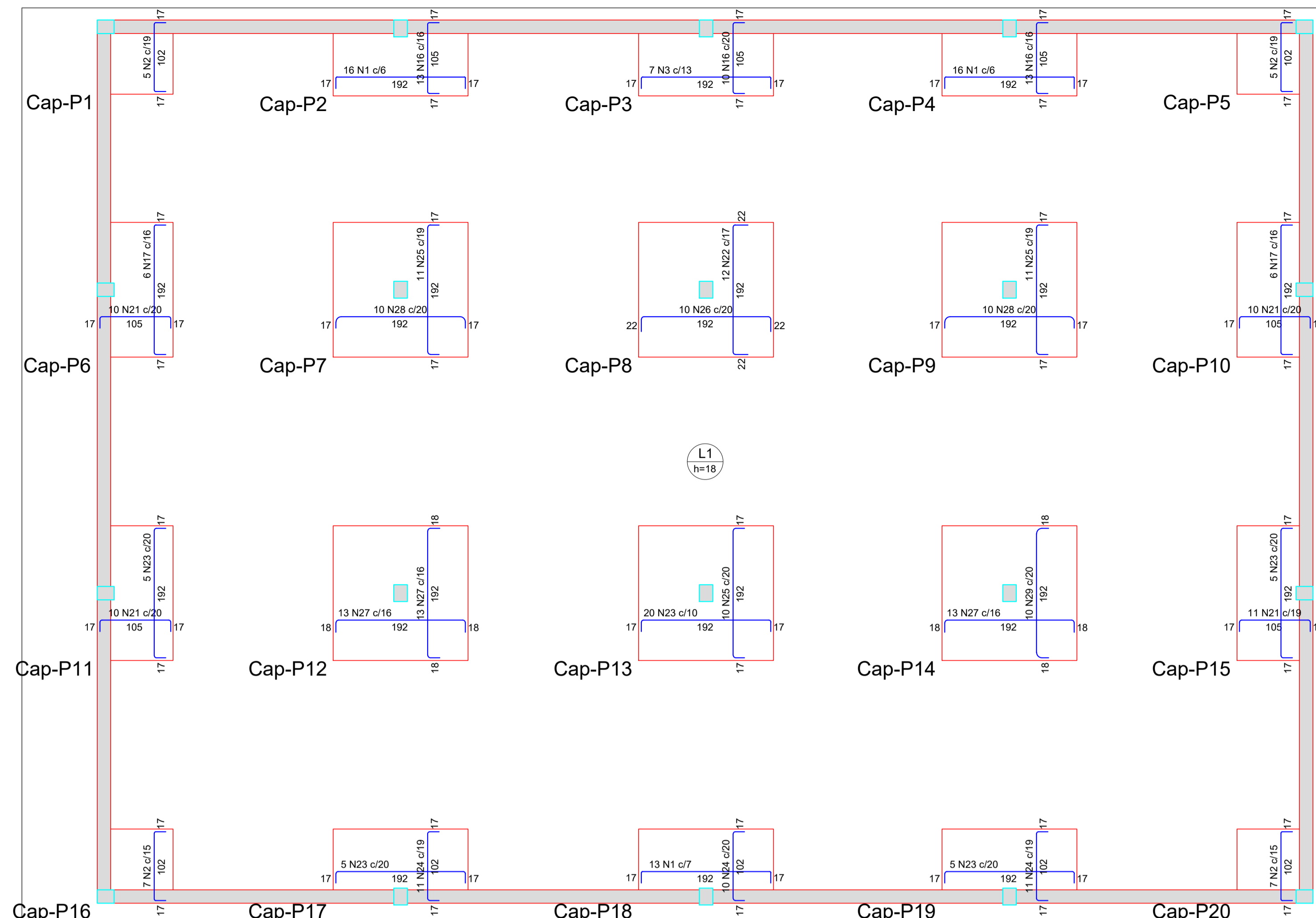
Armação negativa das regiões maciças do pavimento LAJE
