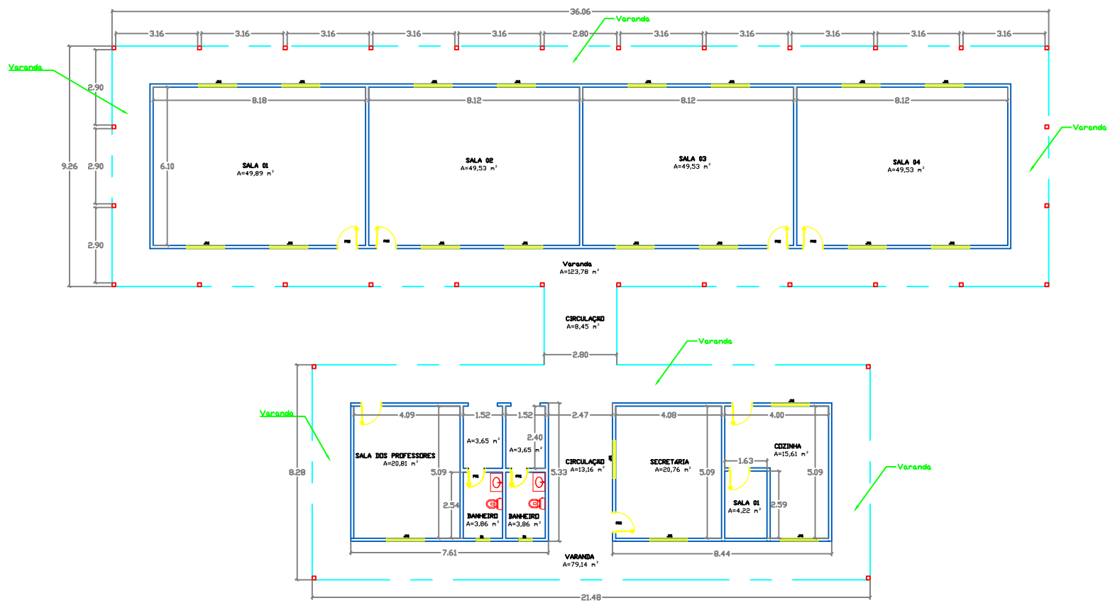
PLANTA BAIXA - ESCOLA ANTIGA ESCALA 1/75
