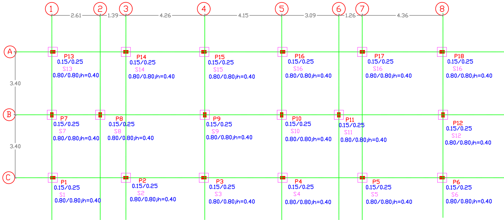
PLANTA DE LOCAÇÃO, SAPATAS E PILARES
