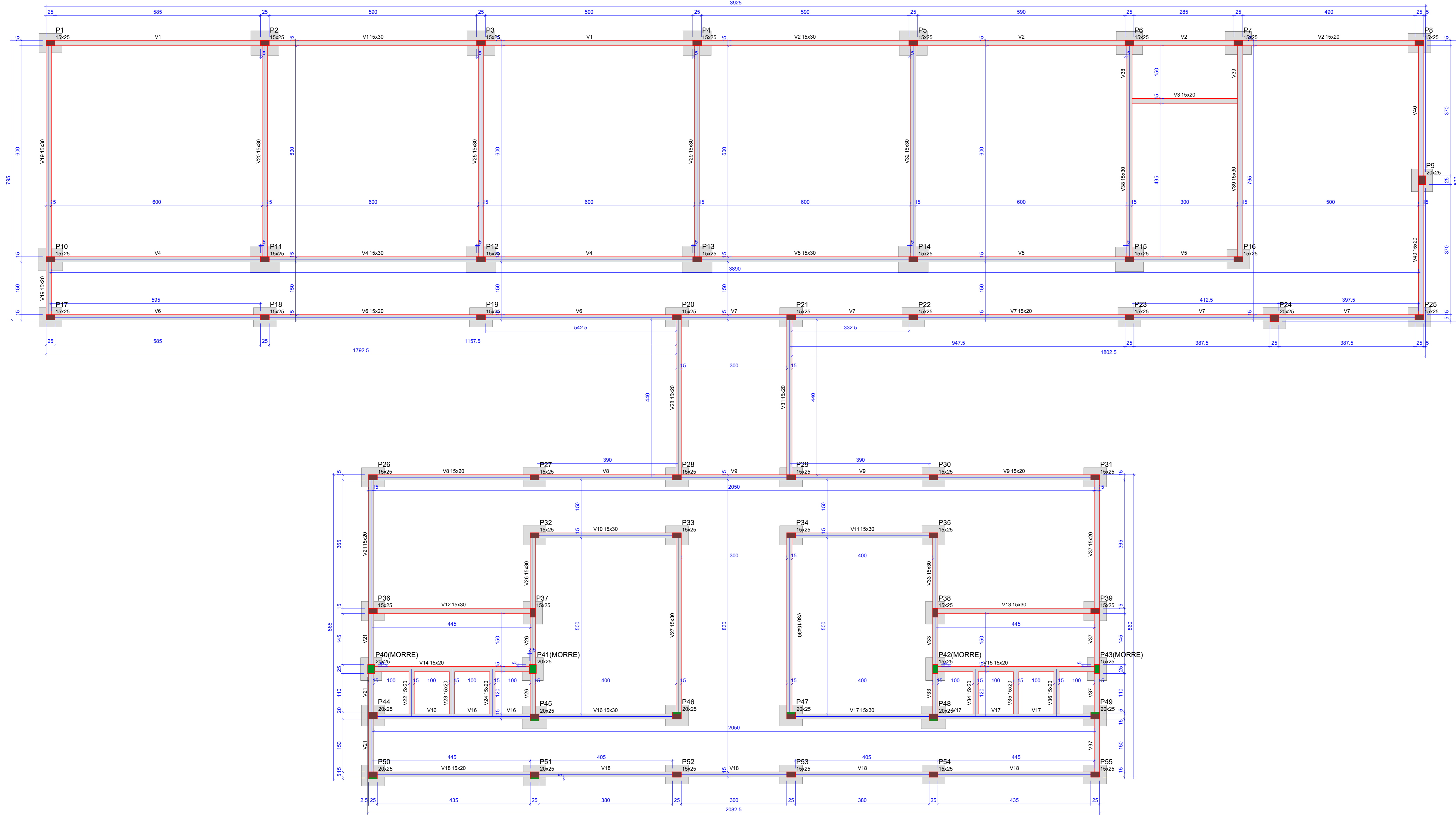
Forma do pavimento FUNDAÇÃO (Nível 0) escala 1:50
