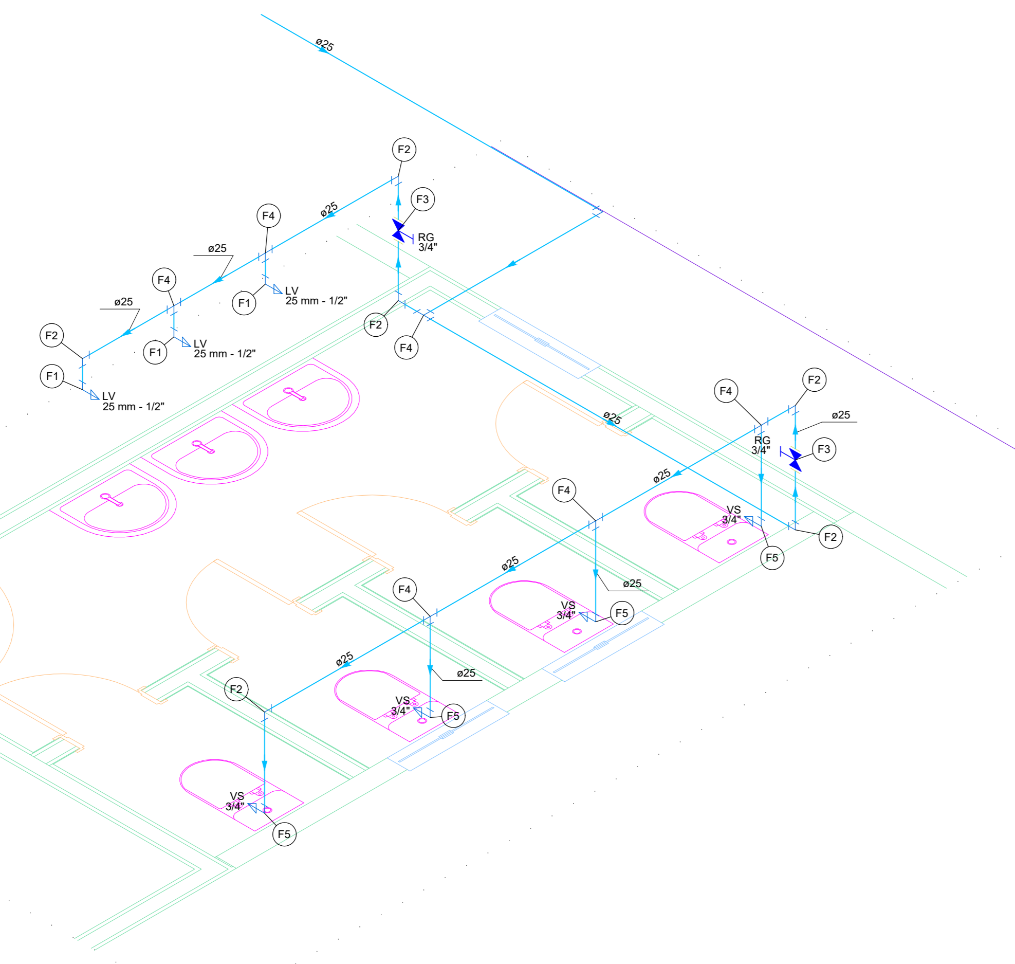
Detalhe HID-2 Escala 1:25
